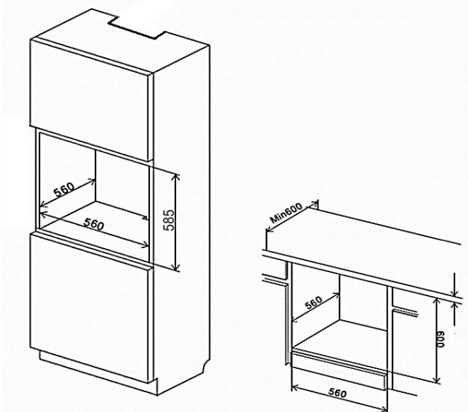
Einbauskizze
