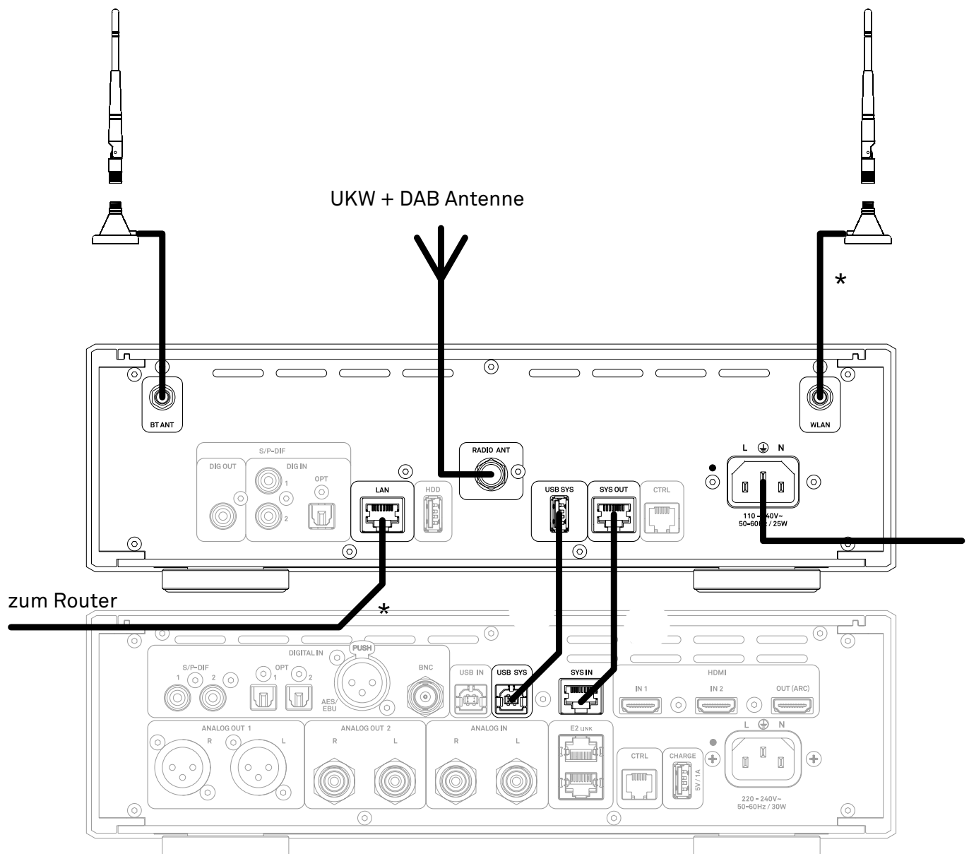
Anschlussschema
