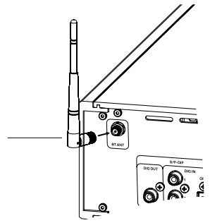
Anschluss der Bluetooth-Antenne
