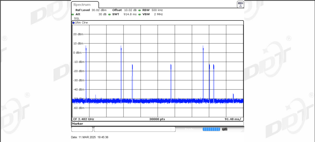
2DH5_Ant1_Hop_2480
