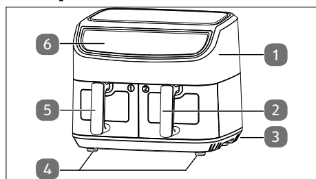
Fig. 1 – Parte delantera
