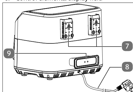
Fig. 2 – Back
