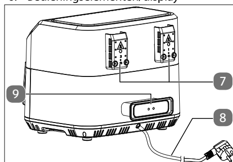
Afb. 2 – Achterkant
