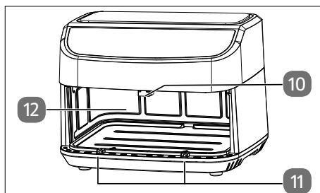
Fig. 3 – Bac à friture
