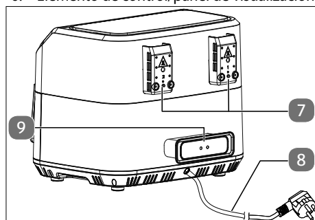
Fig. 2 – Parte trasera
