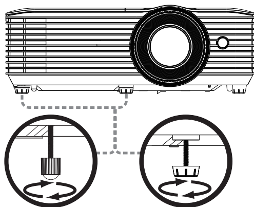
Winkelverstellfüße
