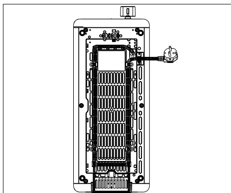
Afb. 5 – Netsnoer opwinden
